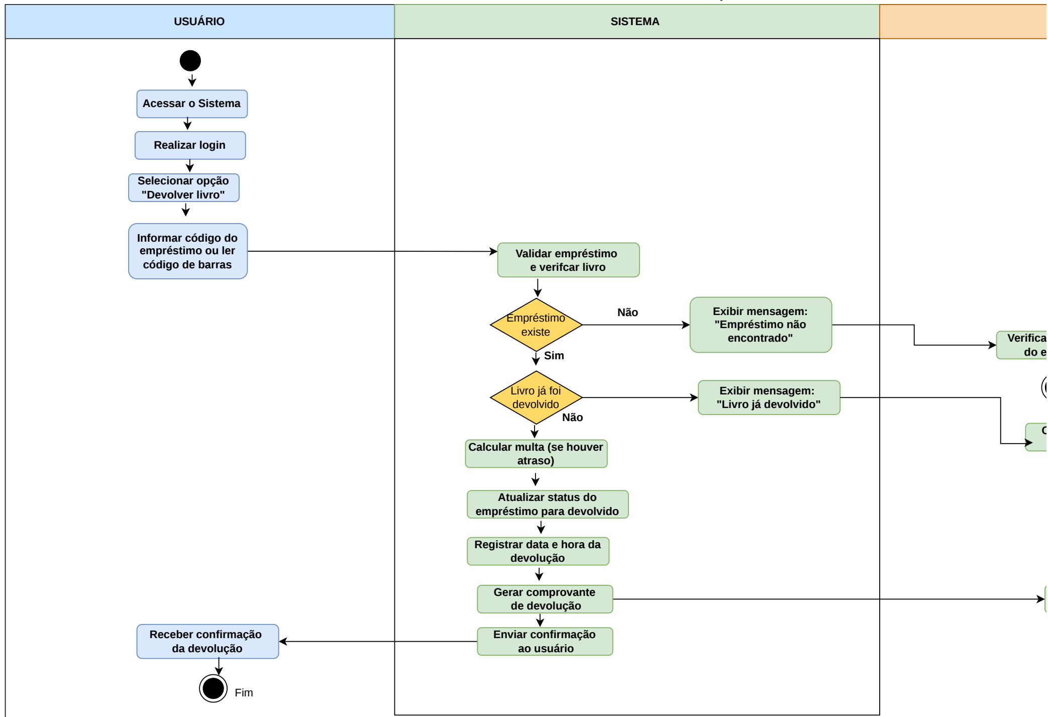
DIAGRAMA DE ATIVIDADES - PROCESSAR DEVOLUÇÃO DE LIVRO
